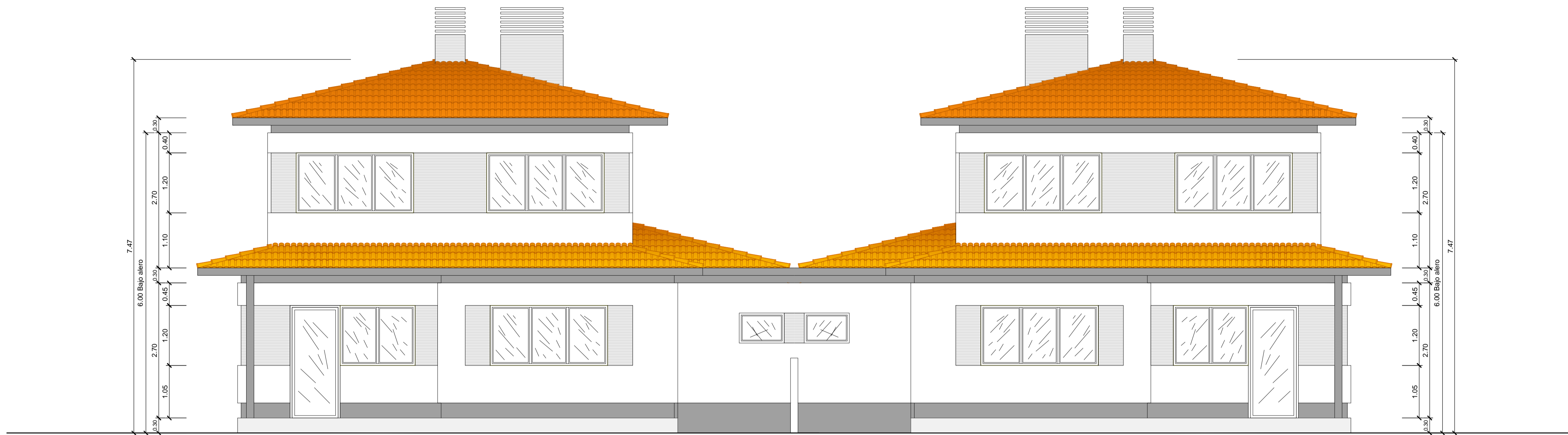
ALZADO TRASERO 3 - 5 - 7
